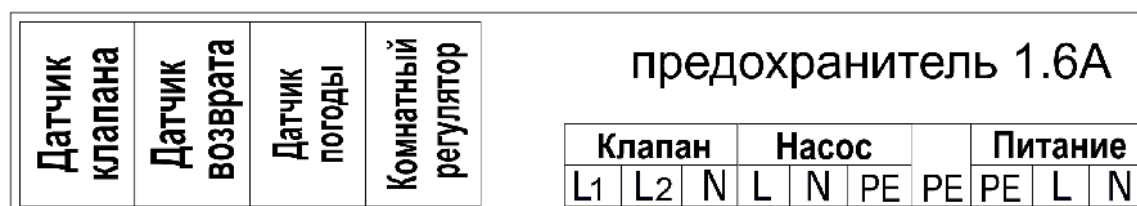
Схема установки
